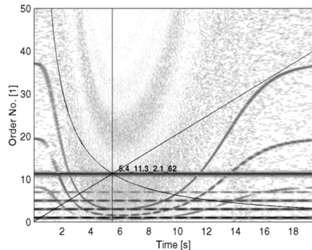
Bild 8: Ordnungsspektrum durch Analyse im Winkelbereich berechnet. Zeitachse durch Interpolation berechnet
