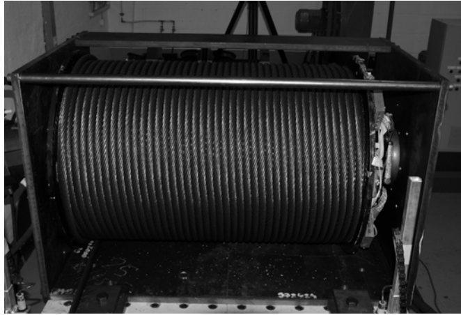
Bild 10: Hybridkonstruktion auf dem Trommelprüfstand
