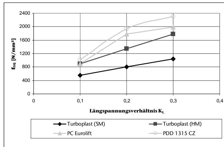
Bild 6: E_{SQ} in Abhängigkeit von k_L ; k_Q = 0,1 ; 1. Lage
